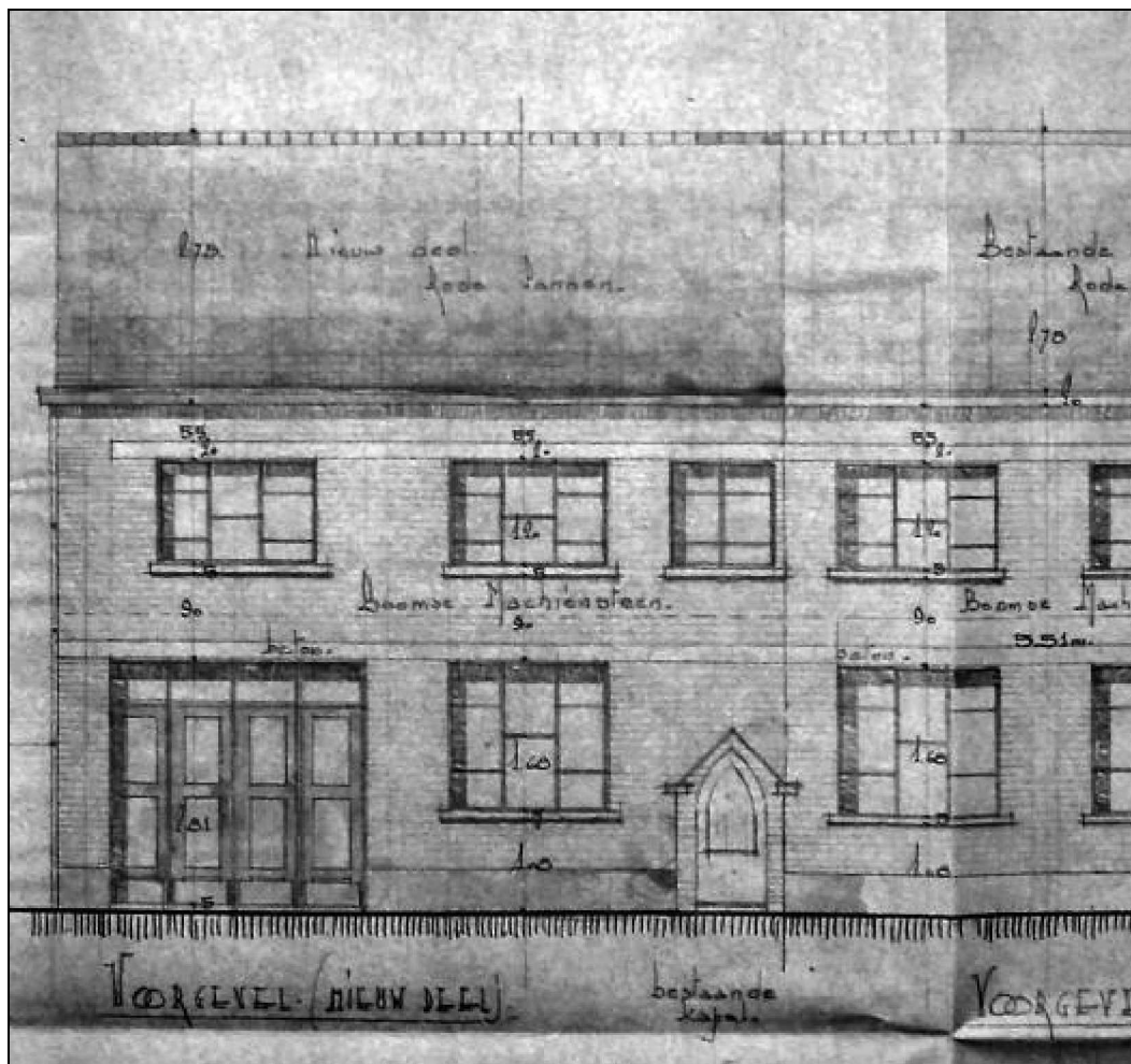
Fragment van het bouwplan voor de vergroting van de schrijnwerkerij Willocx aan de Langeveldstraat (1949, architect Stan. De Smedt). Bron: Gemeentelijk Archief.
